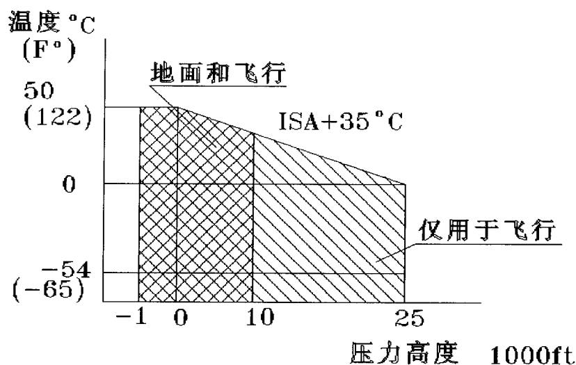
图2 压力高度
