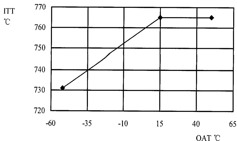
图1 正常起飞ITT限制
