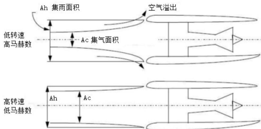
图 33.78-1* 进气系数
