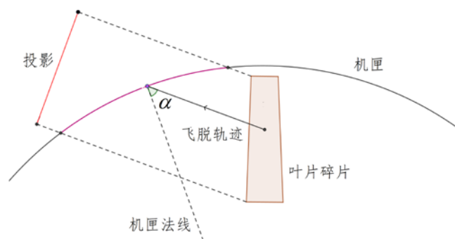
图 33.19-1-1 叶片飞脱轨迹与机匣法线夹角示意图
