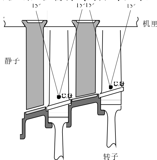
图 33.19-1-2 叶片包容区域定义
