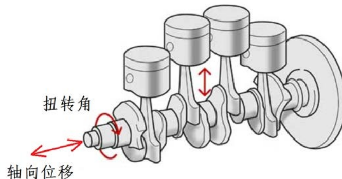
图 33.43-1 轴端位移测量示意
