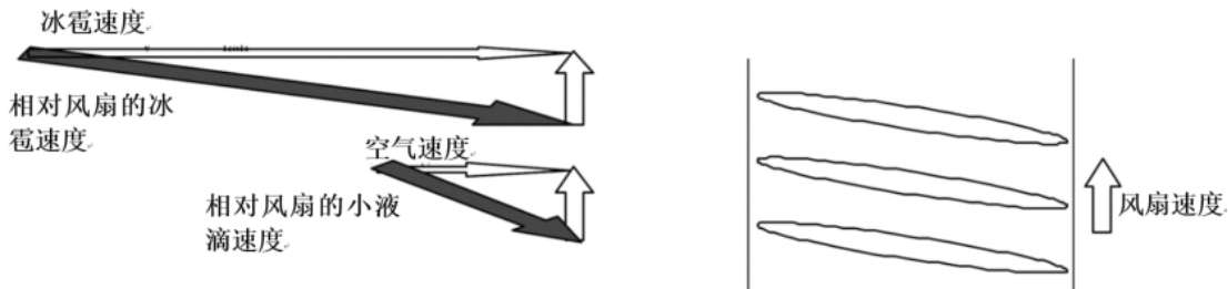
图 33.78-2* 速度矢量图
