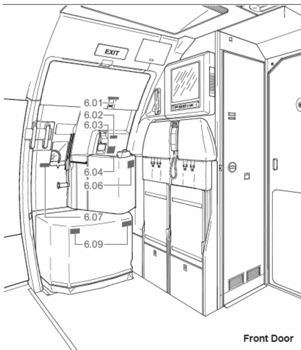
图 31 前部登机门
