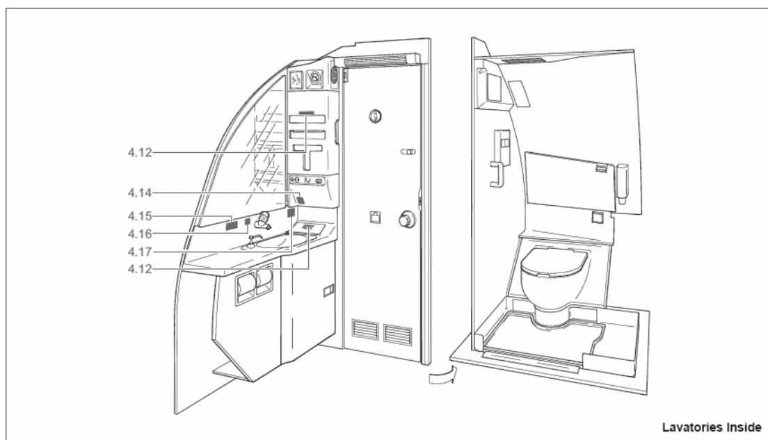
图 21 厕所内部
