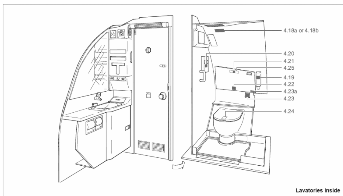
图 22 厕所内部（续）
