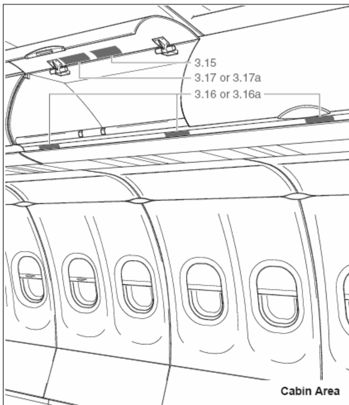
图 15 客舱区域
