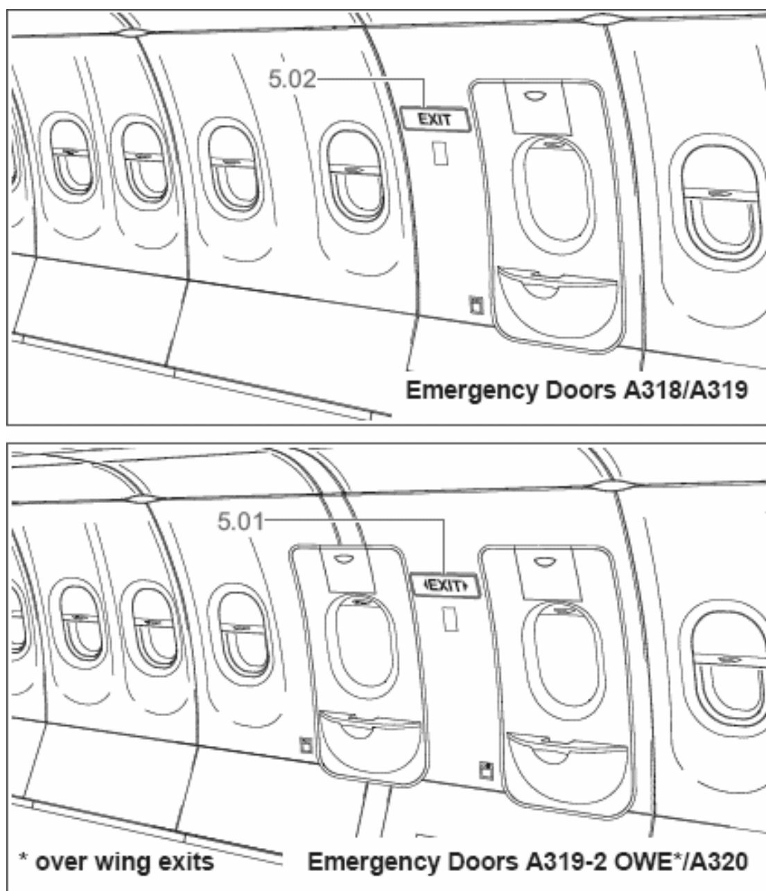
图 25 应急出口
