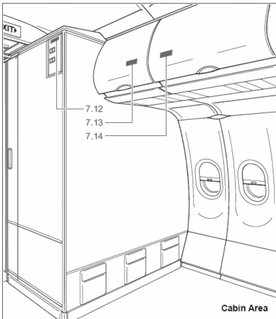
图 44 客舱区域（续）
