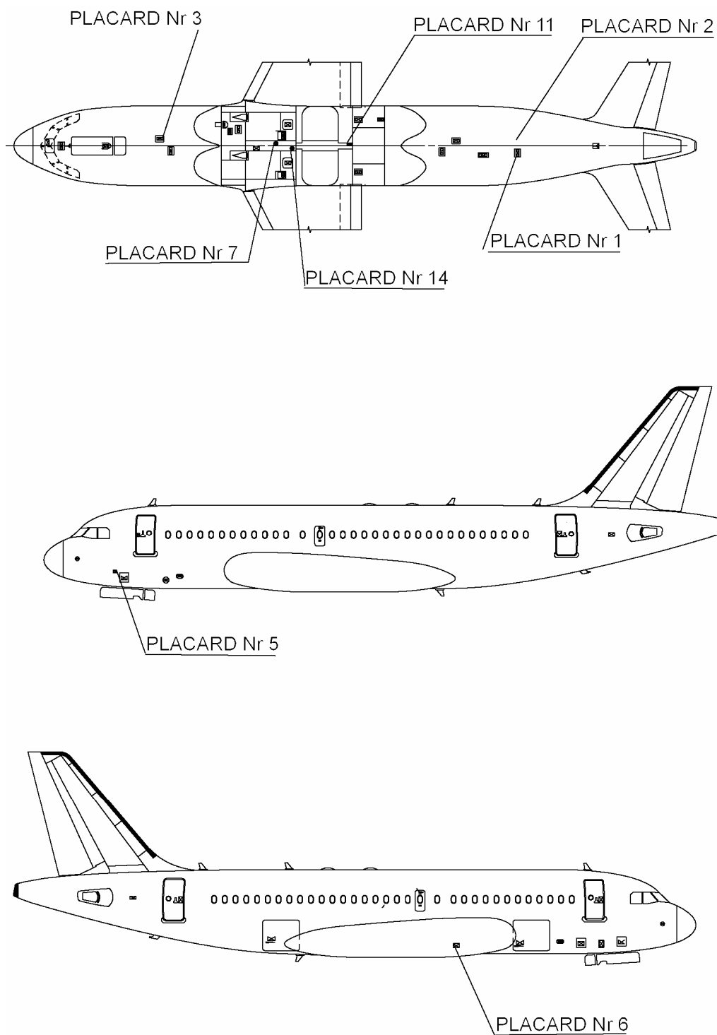
图五 水、燃油
