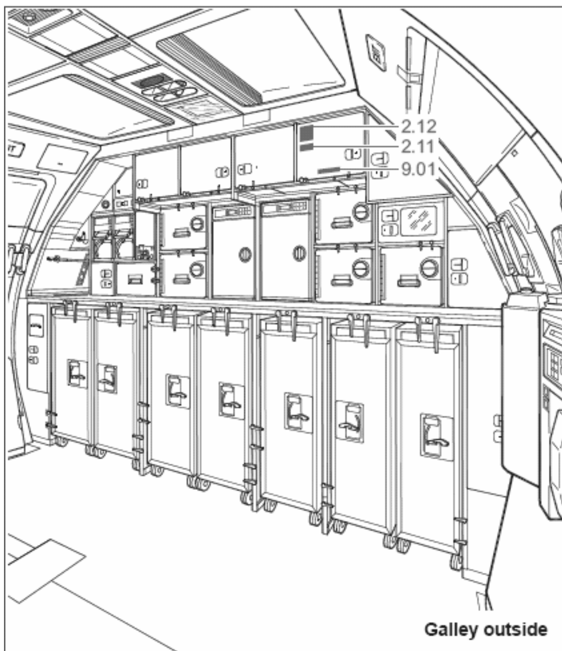
图 52 厨房外部
